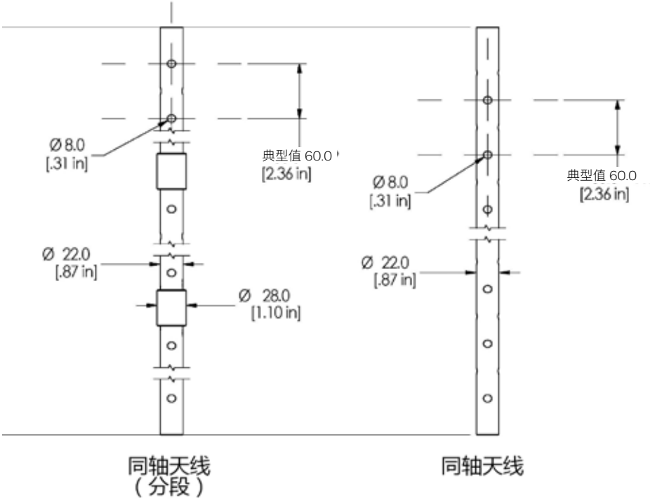
图 26 - SLG720 SmartLine 导波雷达液位计 - 同轴天线
