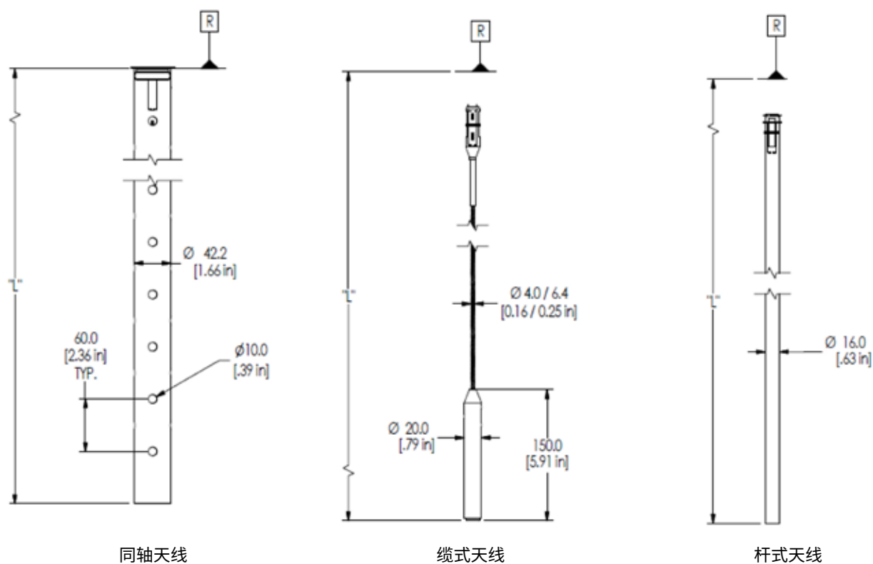
图 30 - SLG726 天线
