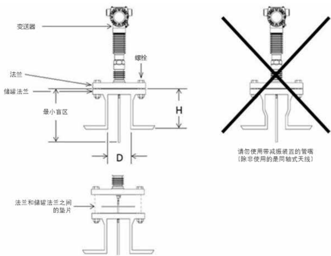
图 13 - 法兰安装
